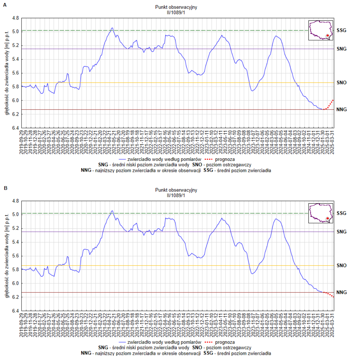
Rys. 15. Prognoza dotycząca stanu wód o zwierciadle swobodnym (gruntowych) na okres 01.03.2025 – 31.03.2025 r. – stacja hydrogeologiczna nr II/1089/1 w miejscowości Turza (woj. podkarpackie). A – prognoza przy założeniu scenariusza A; B – prognoza przy założeniu scenariusza B
