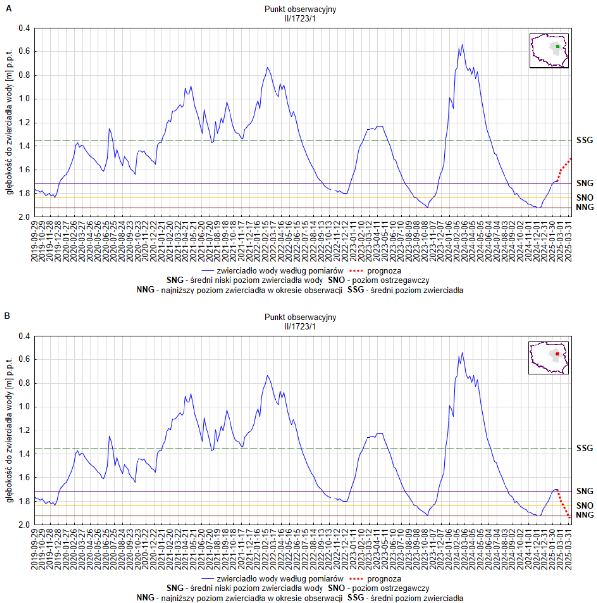
Rys. 12. Prognoza dotycząca stanu wód o zwierciadle swobodnym (gruntowych) na okres 01.03.2025 – 31.03.2025 r. – stacja hydrogeologiczna nr II/1723/1 w miejscowości Kaliska (woj. mazowieckie). A – prognoza przy założeniu scenariusza A; B – prognoza przy założeniu scenariusza B
